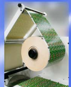
600mm Rewind
